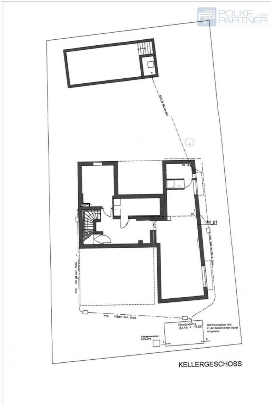
Plan Keller
