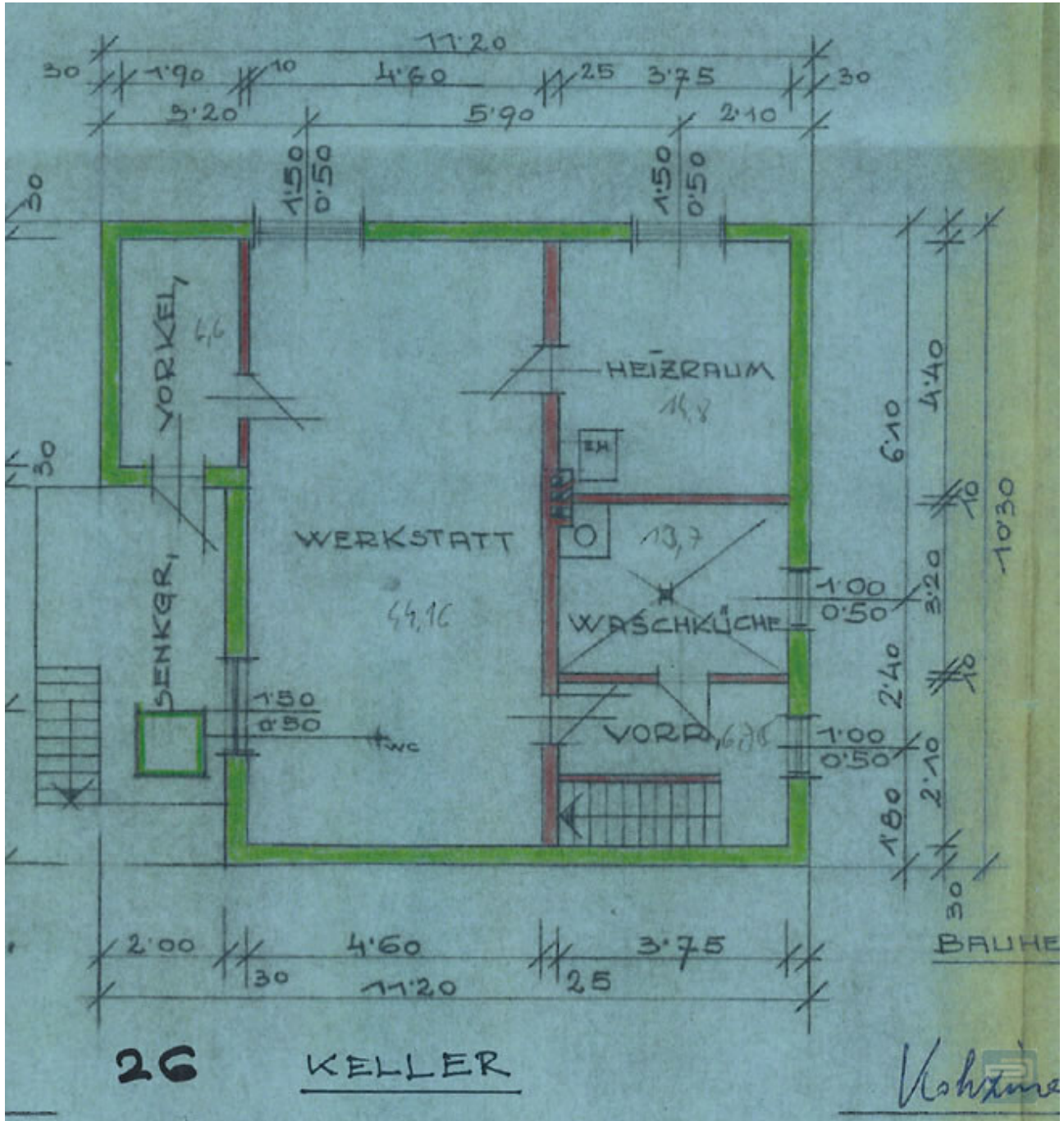
Grundriss Kellergeschoss
