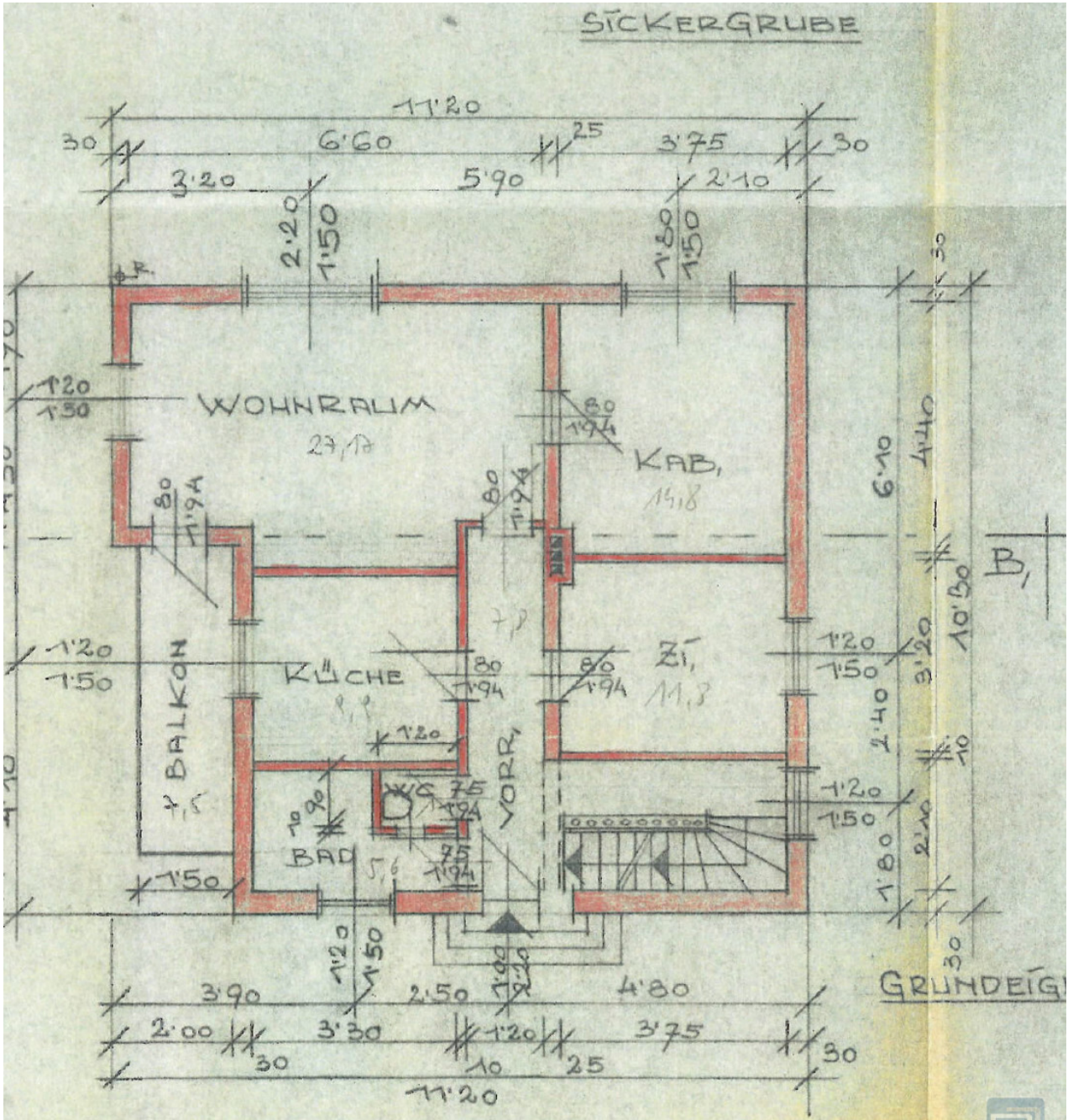
Grundriss Erdgeschoss
