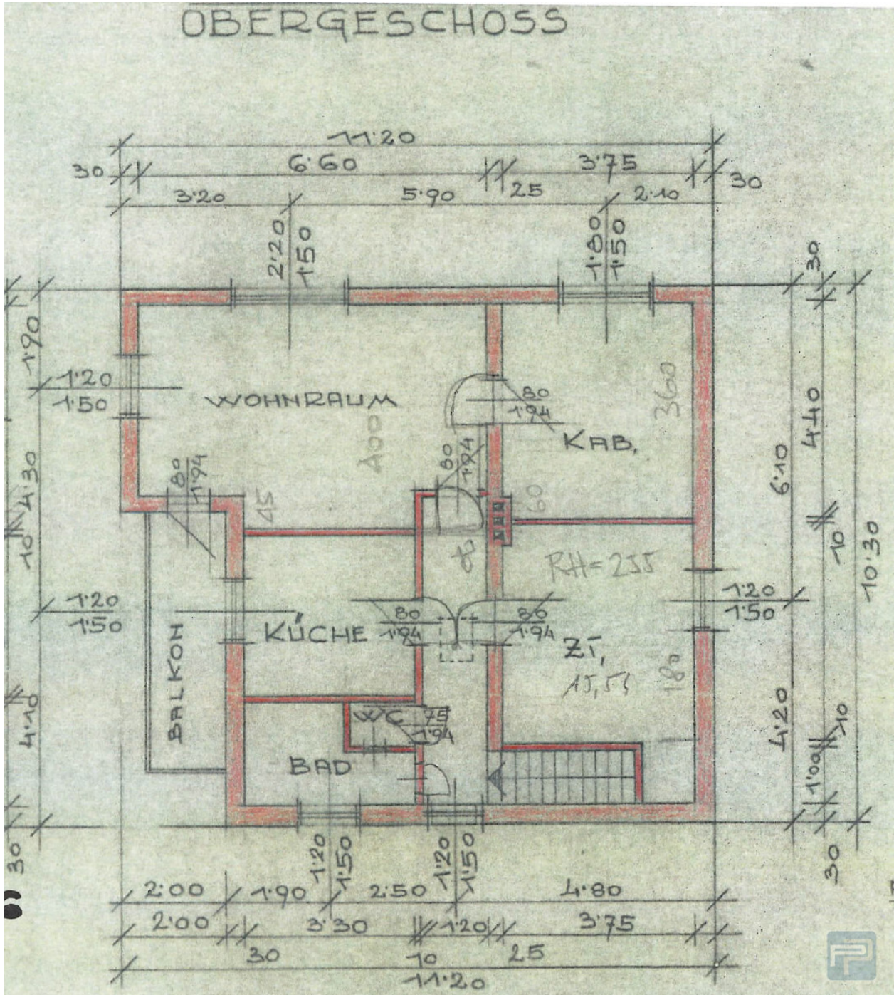
Grundriss Obergeschoss
