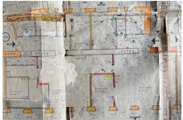
Grundriss
